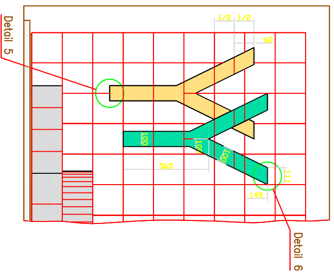
Vermassung B 1 : 10
