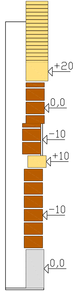
Schnitt B-B
